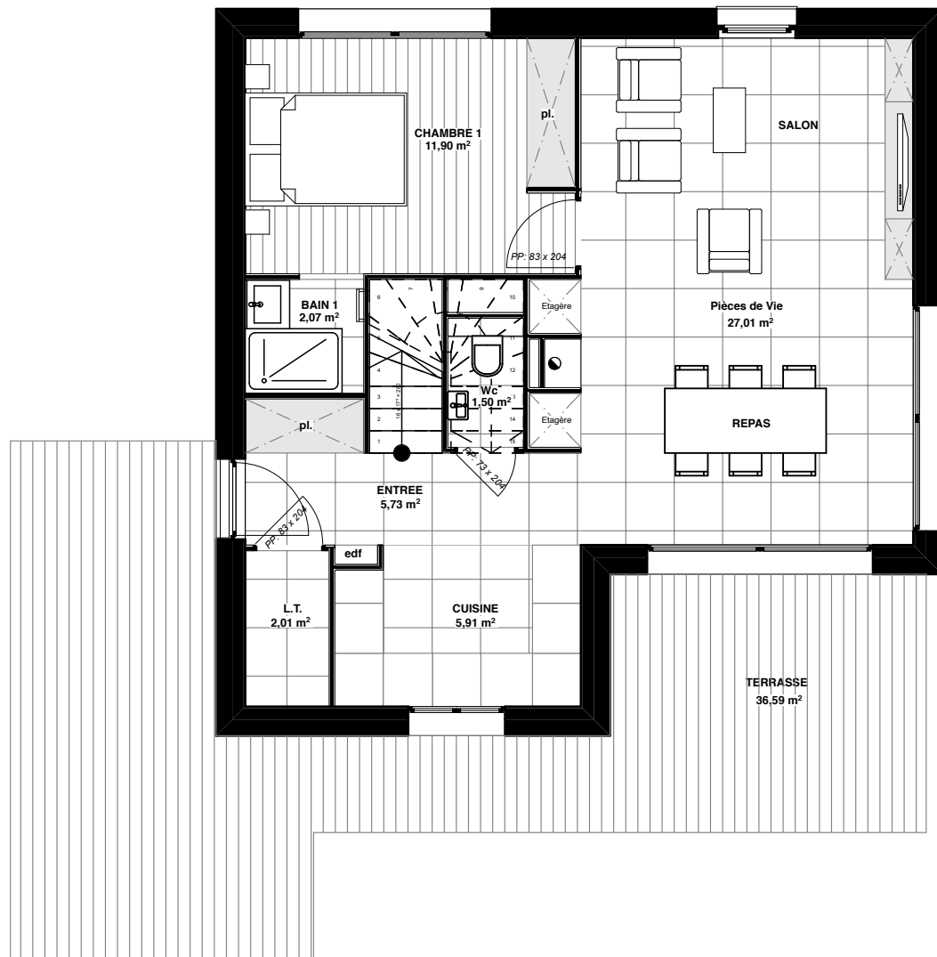
REZ-DE-CHAUSSEE
